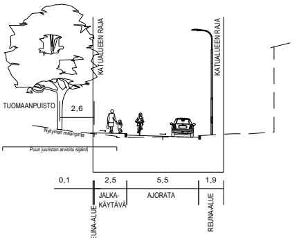
Tuomaankatu (B-B) 1:200
