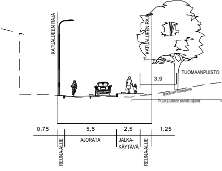
Toivonkatu (A-A) 1:200
